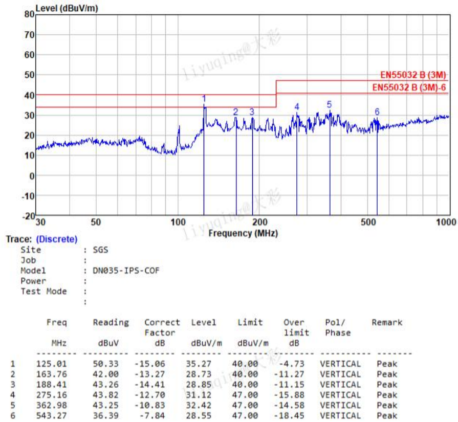
图 6-8 辐射测试垂直方向
